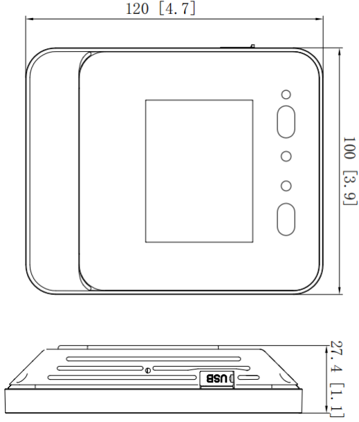
Cihaz Ölçüleri (mm)
