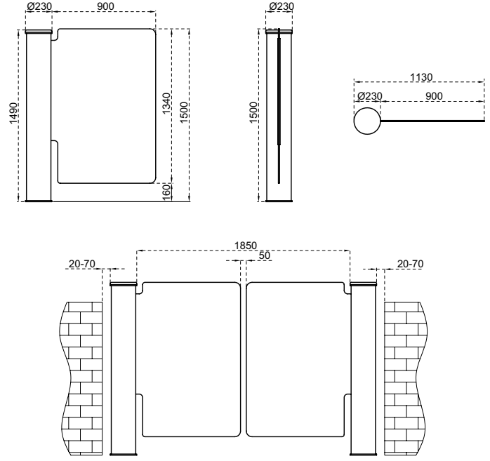
Ölçüler (mm)
