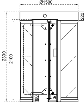
Ölçüler (mm)
